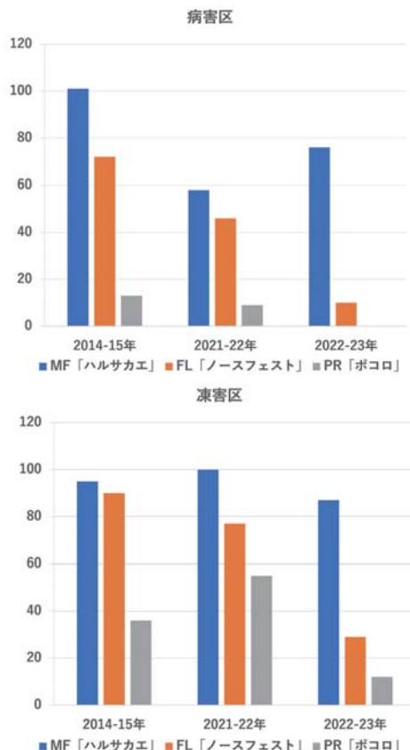
図2 耐寒性特性検定試験における1番草の乾物収量（対照区に対する指数、%） MF：メドウフェスク、FL：フェストロリウム、PR：ペレニアルライグラス
