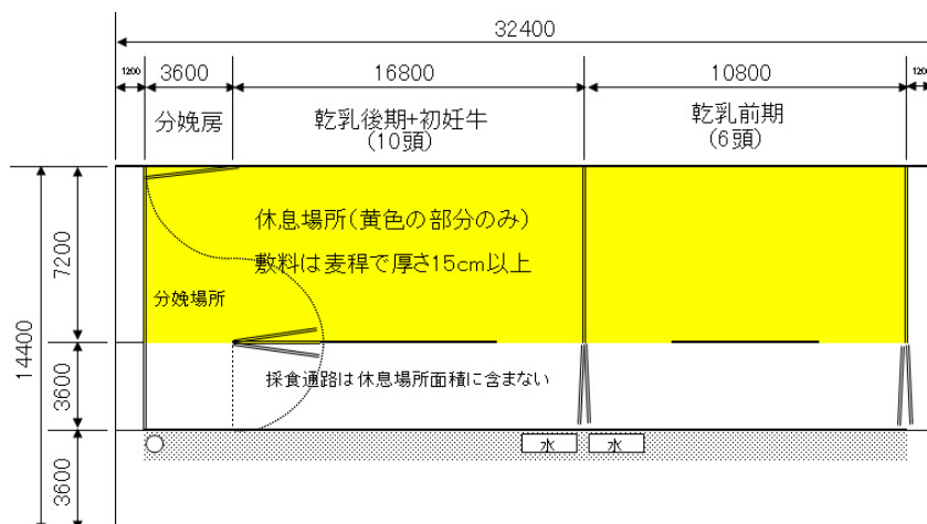
図1. 乾乳・分娩施設の設計例
